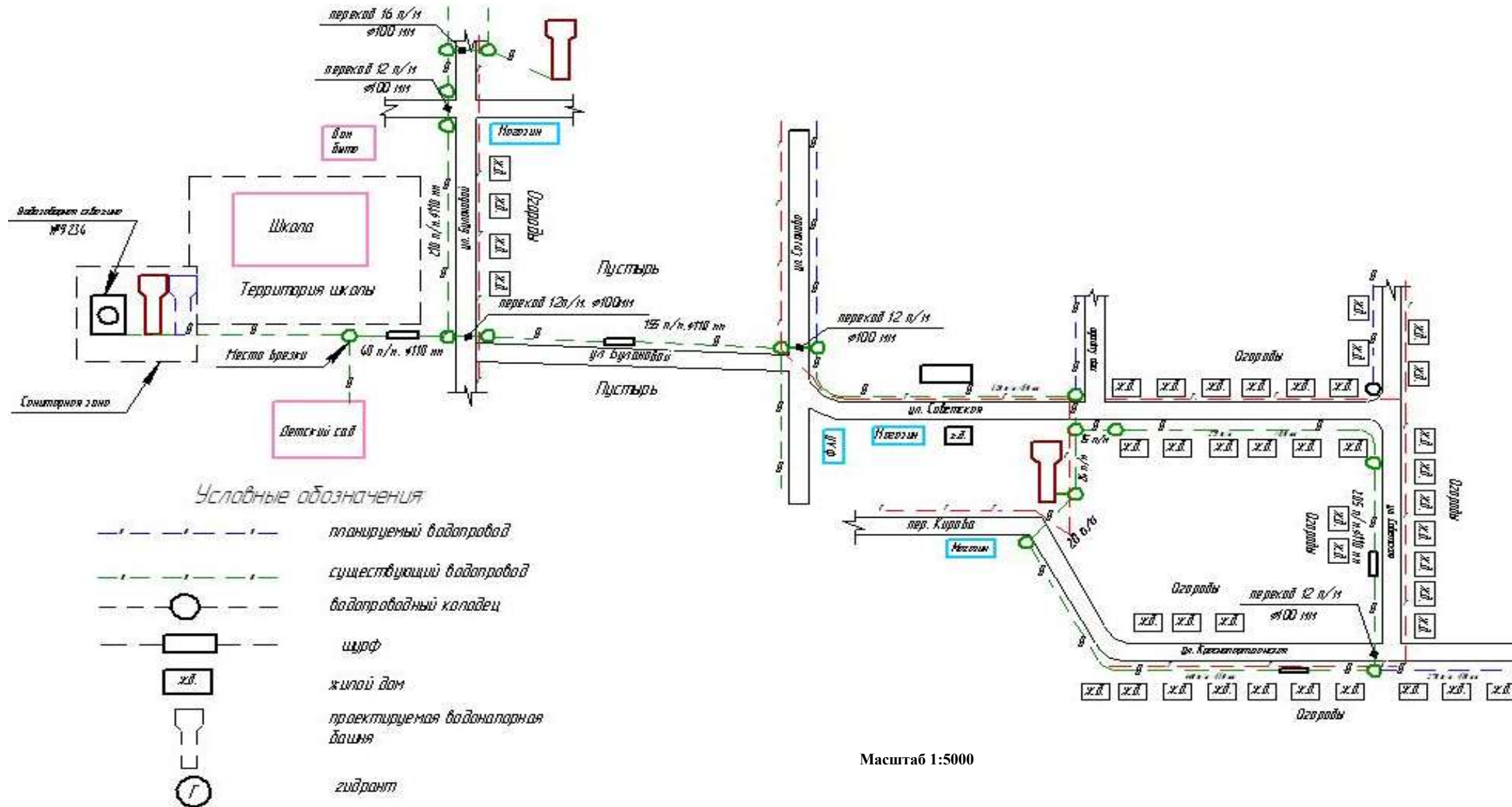
Приложение 24 Схема водоснабжения сл. Кутейниково (ул. Булановой/ул. Советская/ул. Краснопартизанская/пер. Сазонова/пер. Кирова)
